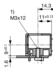
1) Selbstschneide-Schraube
